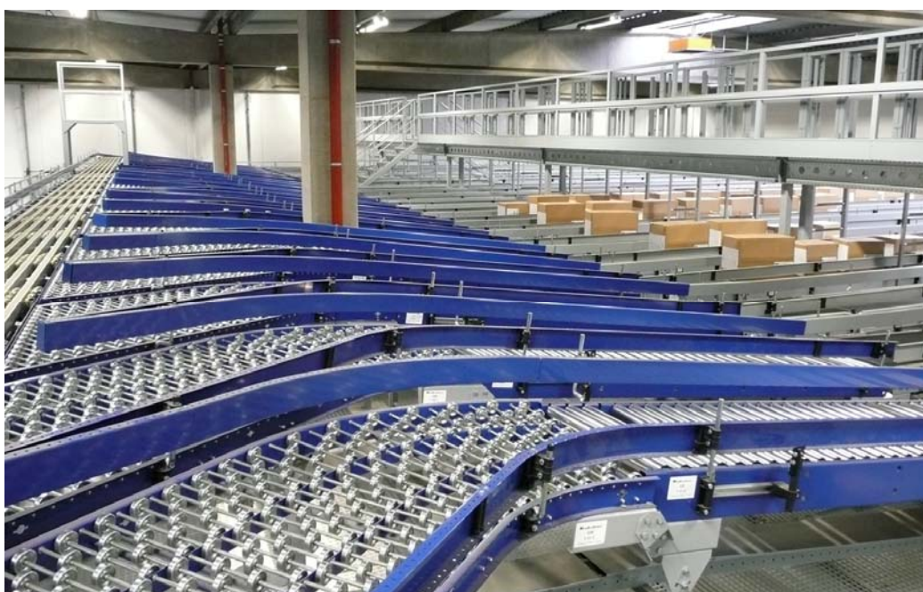
Schenker A/S' nye cross docking-anlæg i Kolding under en prøvekørsel. Klik på billederne for at downloade dem i høj opløsning (2MB)!
